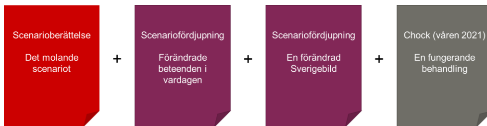
Figur 3: Exempel på ett möjligt scenario. Scenariorättelsen "det molande scenariot" kombineras med två fördjupningar, "förändrade beteenden i vardagen" och "en förändrad Sverigebild", samt med chocken "en fungerande behandling" som antas inträffa under våren 2021.
