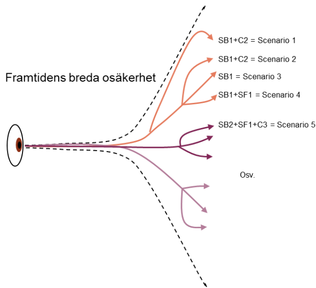
Figur 2: Illustration över hur olika sätt att kombinera scenariorättelser (SB) med scenariefördjupningar (SF) och chocker (C) innebär möjligheter att utforska en bredare framtida osäkerhet. Chocker kan introduceras vid olika tidpunkter i en scenariorättelse vilket illustreras med skilda scenarier 1 och 2. Observera att illustrationen inte är skalenlig och därmed inte säger något om hur stor del av den framtida osäkerheten som täcks in med scenarier – världen är så pass komplex att antalet möjliga framtida tillstånd är nära nog oändligt.
