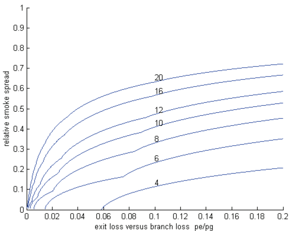
Figur 4.9 Relativ spridning som funktion av tryckfallskvoten \Delta p_e / \Delta p_g och våningsplan.
