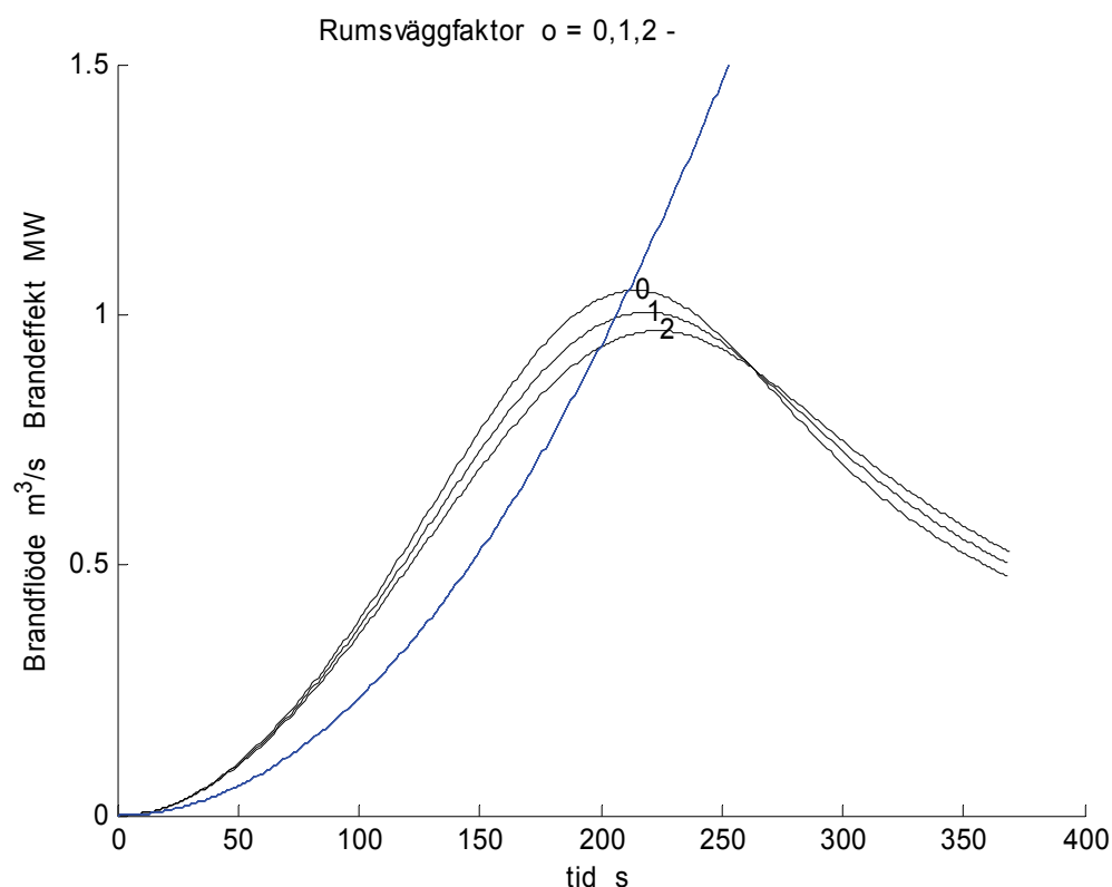
Figur 3.35 Brandflöde och brandeffekt för olika rumsväggfaktor \sigma = 0, 1 och 2 .
