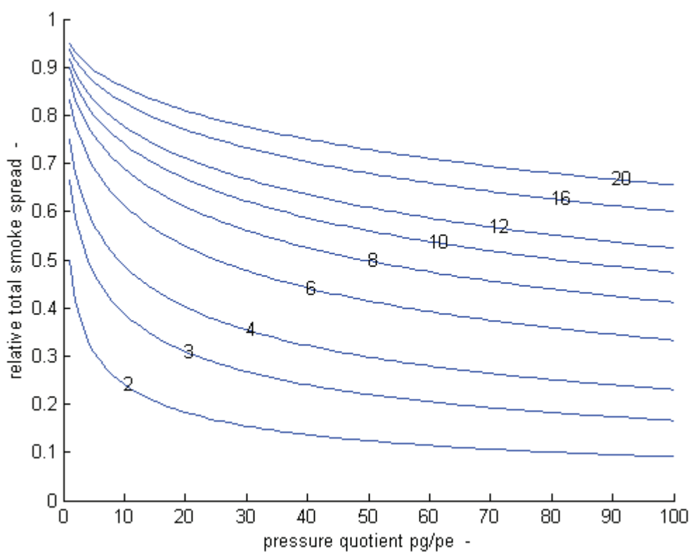
Figur 4.3 Relativ total rumsspridningsandel till alla övriga rum s_i enligt (4.7) som funktion av tryckfallsförhållande f och olika antal rum n = 2, 3, 4, 6, 8, 10, 12, 16 och 20 .
