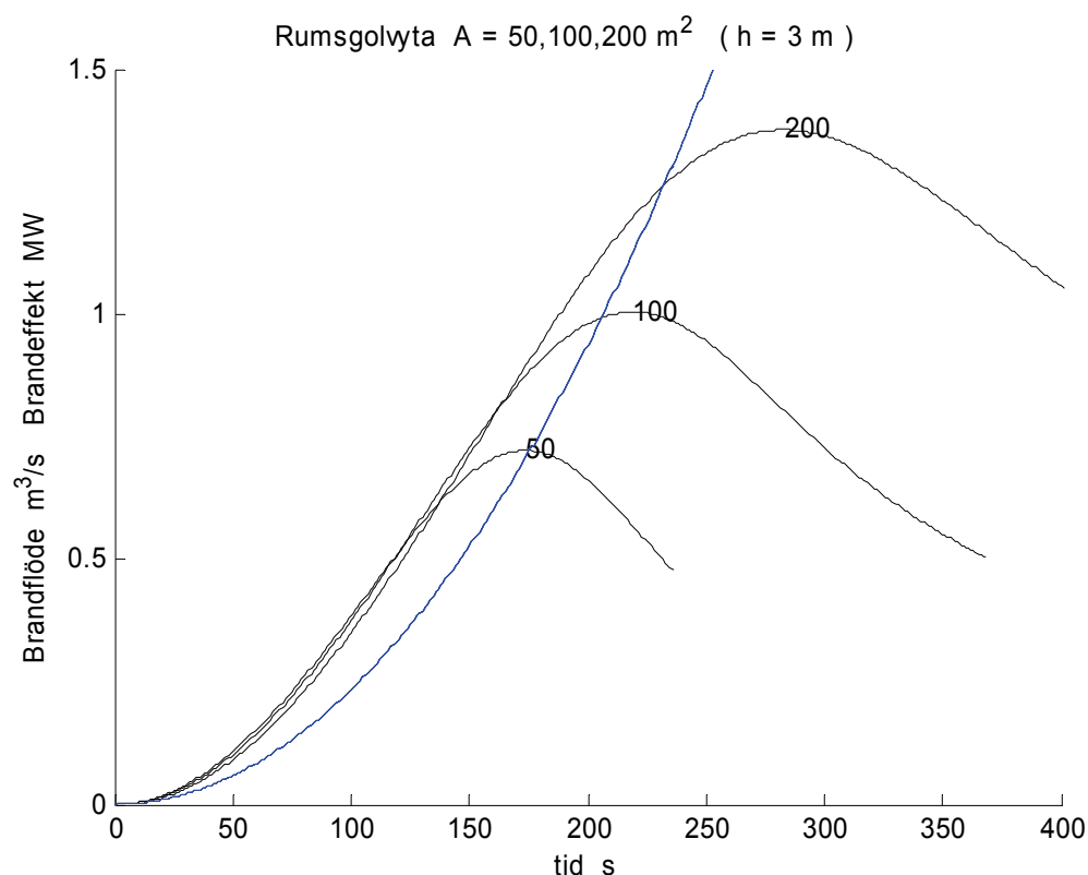
Figur 3.33 Brandflöde och brandeffekt för olika rumsgolvvyta A = 50, 100 och 200 \text{ m}^2 .
