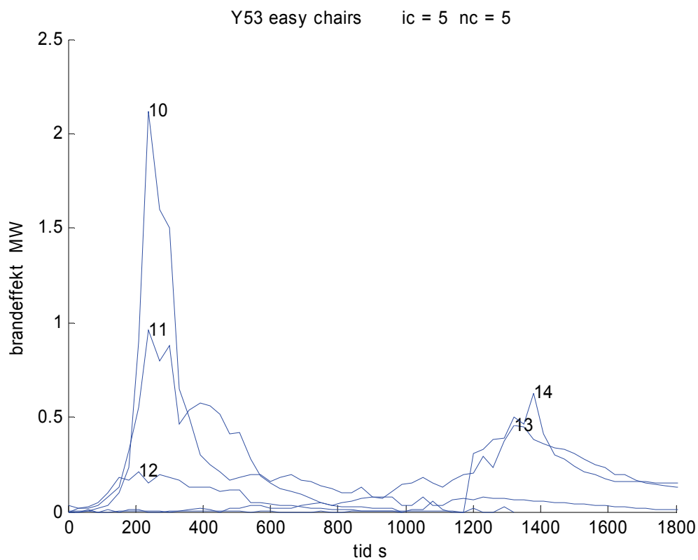
Figur 3.14 Brandeffekt som funktion av tid för olika föremål.
