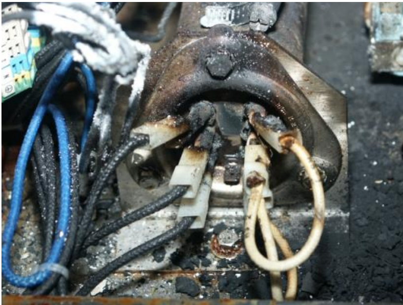
Anslutningar till värmepatronen uppvisar kolningskador.
