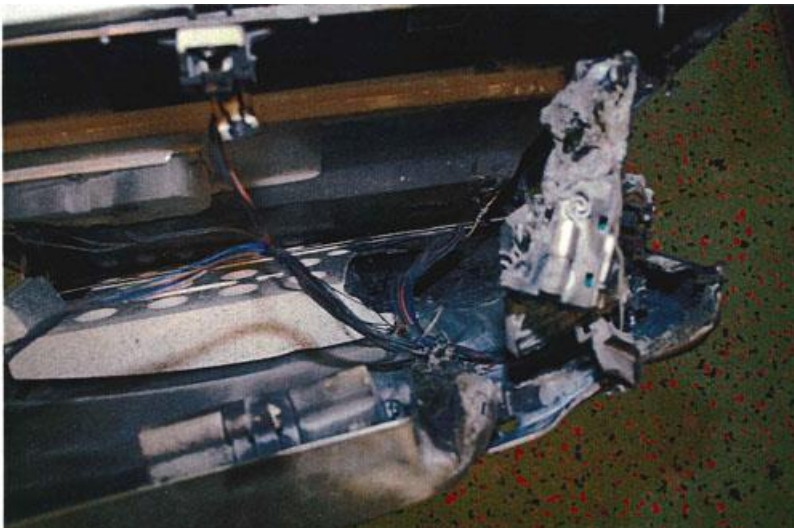
Bild 2. Frontluckans innanmäte med delvis brunnen cellplastisolering.
