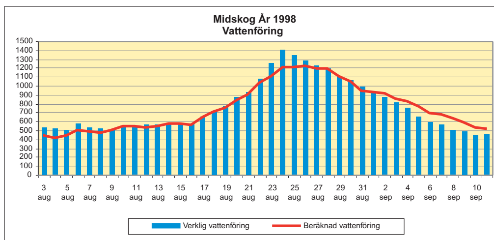
Figur 2. Vattenståndet i Storsjön, tappningen vid utloppet i Hissmofors och flödet i Midskog i augusti 1998 samt den beräknade utvecklingen om vattendomen inte hade ändrats 1988. "DG" är Storsjöns dämningens grän.
