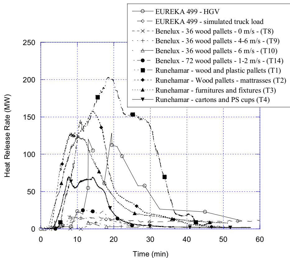
Figur 3.1 Uppmätta brandeffekter hos långträdare i olika fullskaleserier [1, 3, 14].
