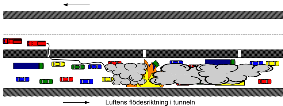
Figur 6.1 Exempel på en räddningsinsats vid en brand i en dubbelrörstunnel med ett tvärsnitt på 90 \text{ m}^2 . Tunnel är utrustad med längsventilation och flödesriktningen är den samma som trafikriktningen. Tunneln är utförd med tvärgående förbindelsevägar mellan de två tunnelrören var 150:e meter och branden antas inträffa utanför en sådan förbindelseväg.
