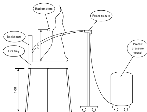
Figur 1. Principskiss av försöksutrustning och uppställning enligt SP Metod 2580 vilken legat till grund för genomförda försök. Skissen visar mjuk påföring via en backboard (gentle application). Vid direktpåföring (forceful application) används ingen backboard-plåt utan skumstrålen riktas direkt mot bränsleytan.
