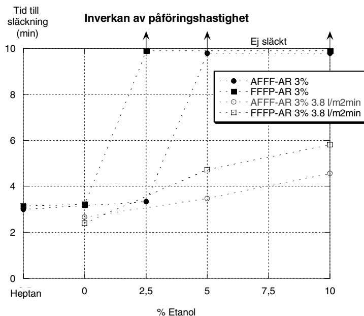
Figur 3 Tid till total släckning som funktion av bränslesammansättning med fördubblad påföringshastighet (3,8 l/m 2 min). Referensdata (1,9 l/m 2 min) från Figur 2 redovisade som jämförelse. (Tider redovisade som 10 min avser att släckning ej erhöjts)
