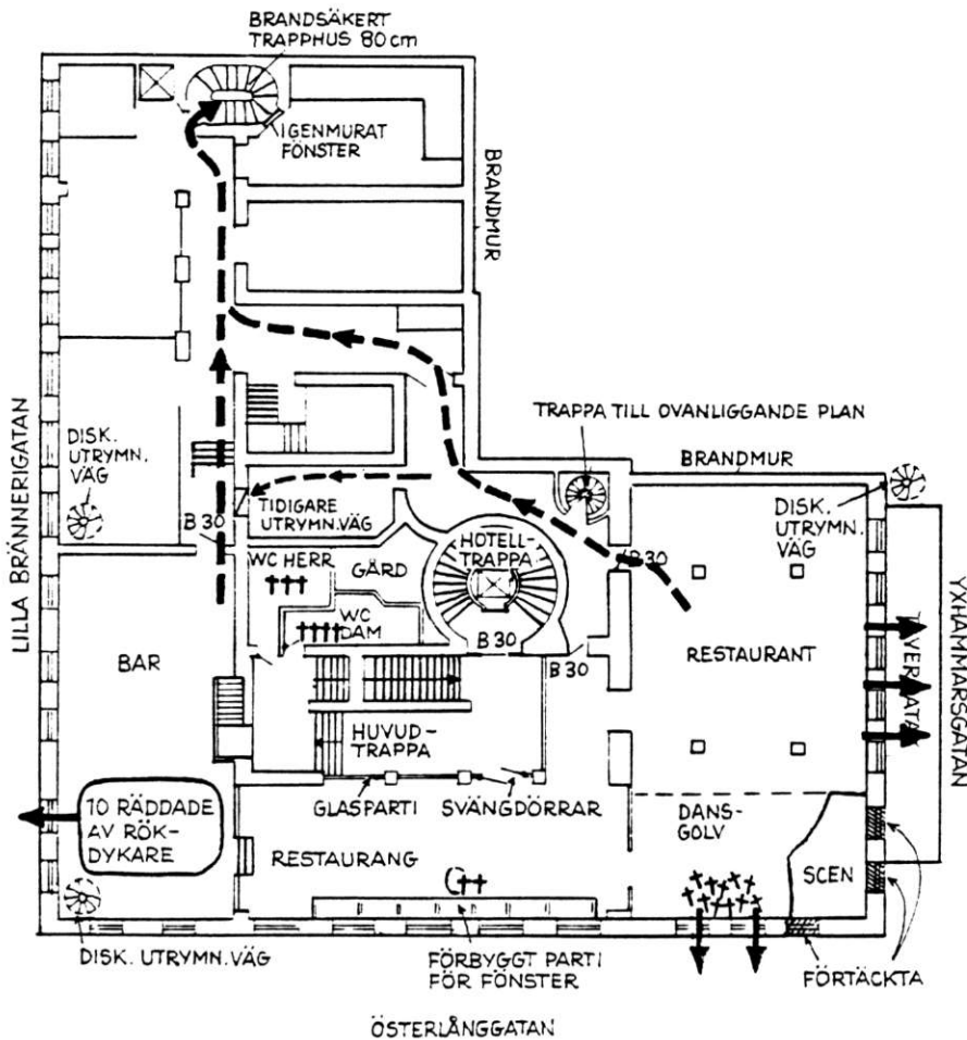
Fig 11 Utrymningsväg genom köket markeras genom steckade pilar. Utrymning via tavernataket och fönster visas med pilar. Plats där offer hittats markeras med kors.
