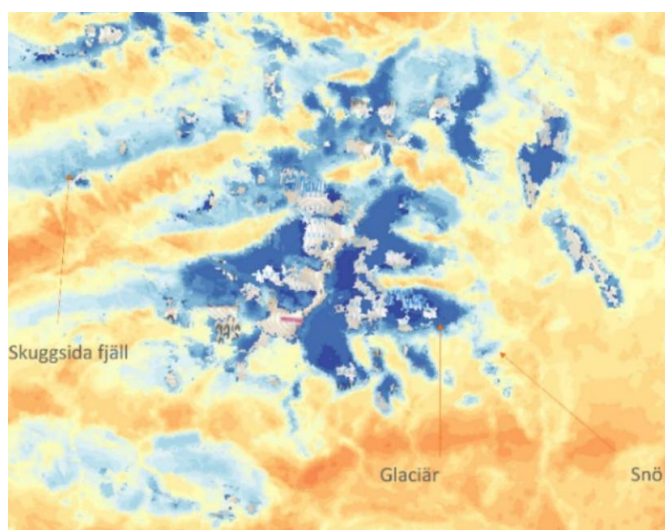
Figur 8. Exempel från Kebnekaiseområdet med svala ytor; glaciär, snö och skuggsidor.
