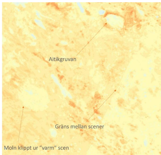
Figur 6. Exempel på bortklippt moln, gräns mellan scener samt hur Aitikgruvan syns i karttjänsten.
