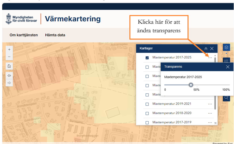
Figur 4. Karttjänst för värmekartering.
