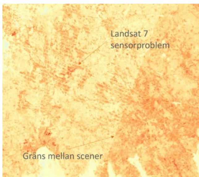
Figur 5. Exempel på artefakter i karttjänsten som visar en gräns mellan scener samt hur ränder uppstår på grund av sensorproblem för Landsat 7.
