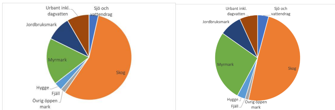
Figur 3. Till vänster: Markanvändning inom Lagans avrinningsområde uppströms Värnamo. Till höger: Markanvändning inom Storåns avrinningsområde, inlopp Bolmen 7 .
