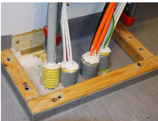
I en brandcellsgräns måste hål eller genomföringar för exempelvis ledningar eller rör brandtätas. Foto: MSB
