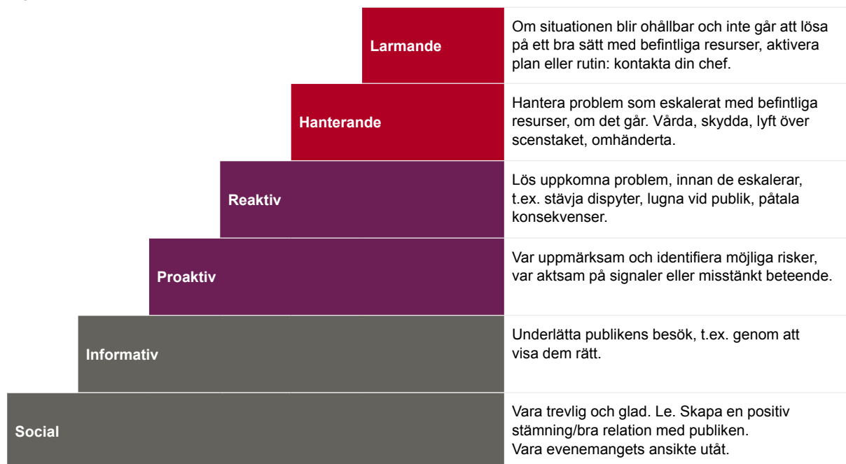
Figur 30. Fokustrappan.
