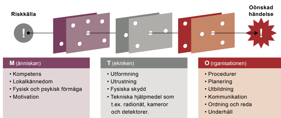
Figur 2. Lökprincipen, MTO-perspektivet.
